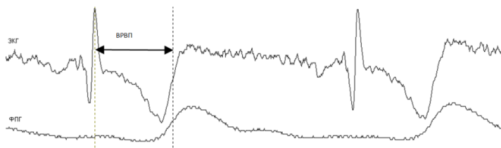
Рис. 1 – Принцип измерения ВРПВ
