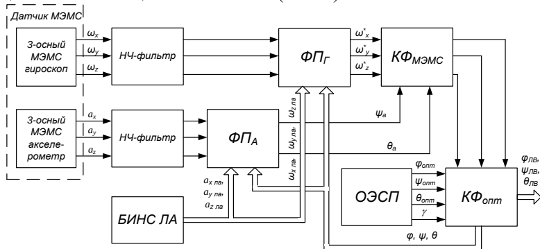
Рис. 1 – Структурная схема разработанной гибридной СП
