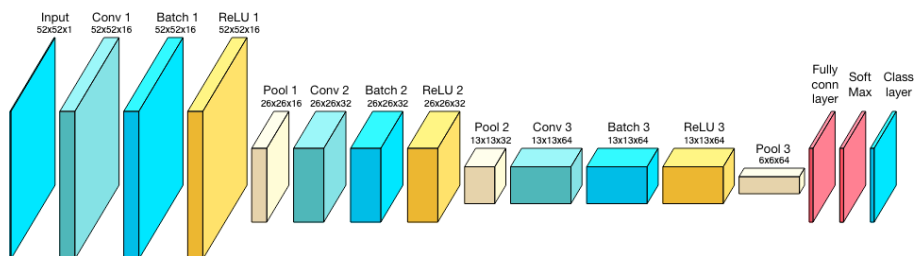
Рис. 1 – Архитектура используемой сверточной сети
