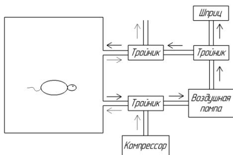
Рис.1 – Схема выполненной экспериментальной установки
