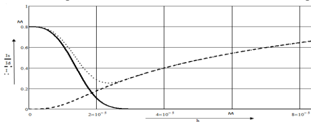
Рис. 1 – Зависимость изменения коэффициентов зеркального (s), диффузного (d) и смешанного отражения от высоты микронеровностей
