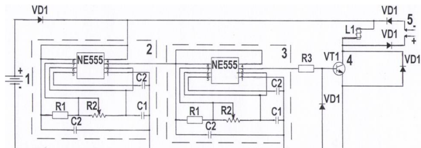
Рис. 2. – Принципиальная схема портативного миостимулятора
