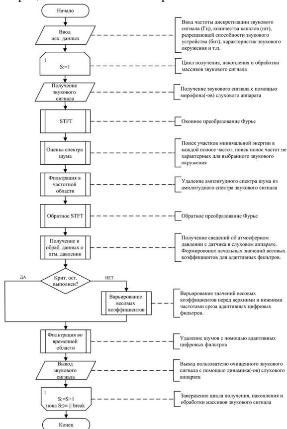
Рис. 1 – Алгоритм адаптивного шумоподавления для слухового аппарата
