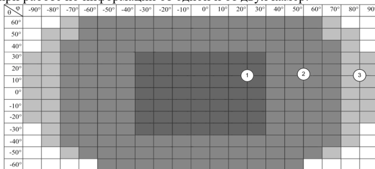
Рис. 3 – Рабочий диапазон углов ОЭСП изделия НСЦИ-В
