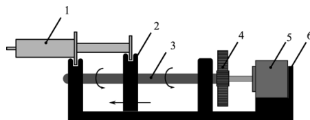
Рис. 1 — Схема шприцевого дозатора: 1 — шприц, 2 — подвижный модуль с внутренней резьбой, 3 — вал с резьбой, 4 — зубчатая передача, 5 — шаговый двигатель, 6 — корпус [5]
