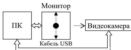
Рис. 1 – Структура аппаратной реализации автоматизированной измерительной системы метрологических испытаний
