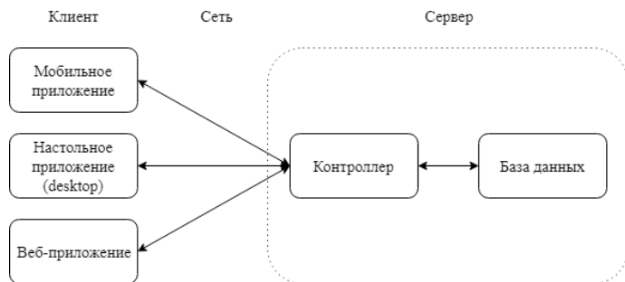
Рис. 1 – Клиент-серверная архитектура приложения
