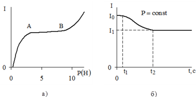
Рис. 1 – а) зависимость силы тока I от величины давления электрода на кожу, б) реакция БАТ на процесс измерения в случае патологии
