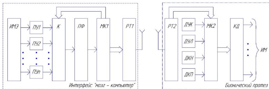
Рис. 1 – Структурная схема системы управления протезом нижней конечности с помощью сигналов мозговой активности
