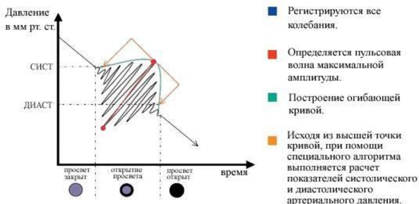
Рис. 1 – Принцип измерения АД осциллометрическим методом
