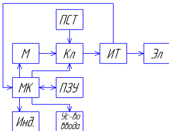
Рис. 1 – Структурная схема разработанного устройства электросон: ИТ-измеритель тока; КЛ-ключ; ПСТ-параметрический стабилизатор тока; М-мультивибратор; Эл-электрод; Инд-индикатор; МК-микроконтроллер; ПЗУ-постоянное запоминающее устройство.
