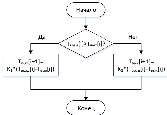
Рис. 1 – Алгоритм вычисления состояния датчика
