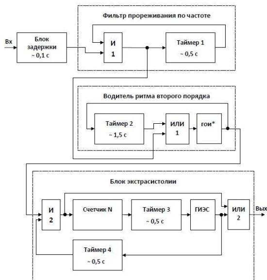
Рис.1 – Структурная электрическая эквивалентная схема АВ - соединения. И, ИЛИ – логические элементы, *ГОИ – генератор одиночных импульсов, ГИЭС - генератор одиночных импульсов «экстрасистолии»
