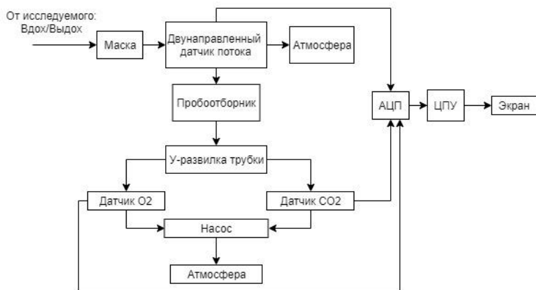
Рис. 1 – Структурная схема аппарата для оценки респираторной системы
