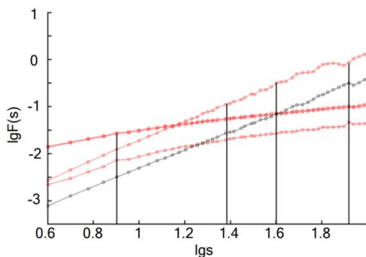
Рис. 1 – Зависимость флуктуационной функции от масштаба для образца без отжига. Наличие нескольких кривых соответствует различным степеням сглаживания метода Scale-Space DFA
