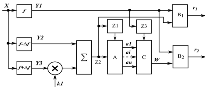
Рис.1 – Структурная схема алгоритма: « f », « f-\Delta f », « f+\Delta f » - узкополосные фильтры; A – блок анализа; Z1 -блок памяти сигнала Z1 ; Z2 -блок памяти сигнала Z2 ; C - блок синтеза; B1 , B2 – блоки вычисления коэффициентов корреляции.
