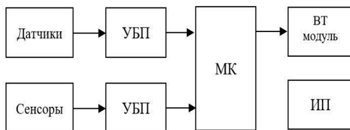
Рис. 1 – Структурная схема носимого устройства регистрации сигналов
