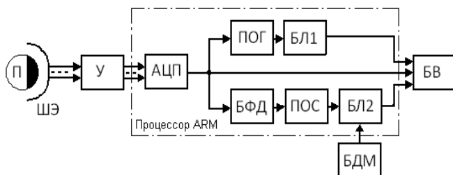
Рис. 1 – Структурная схема скринингующей системы диагностики:
