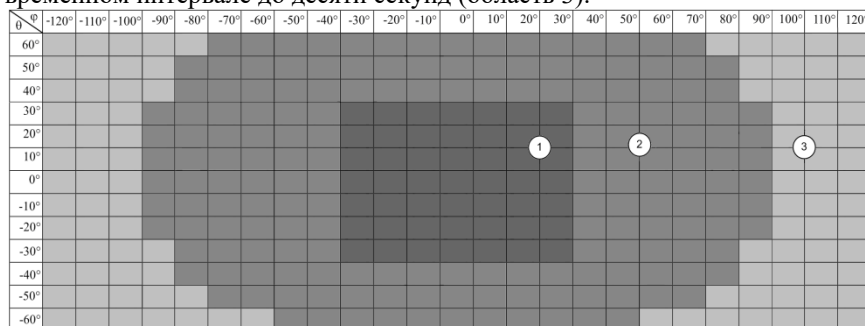
Рис. 4 – Рабочий диапазон углов гибридной СП изделия НСЦИ-В
