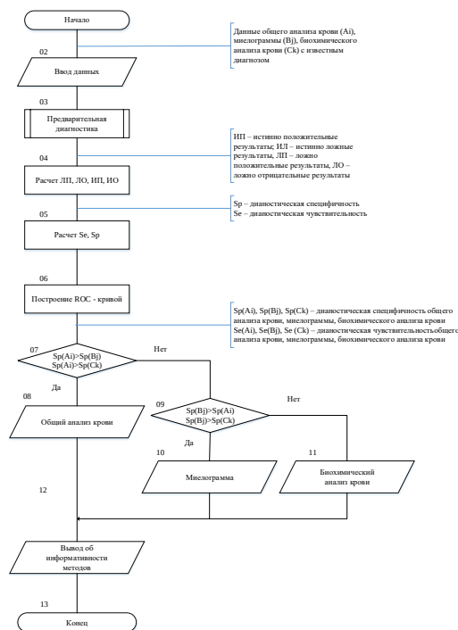
Рис. 1 – Схема графического алгоритма
