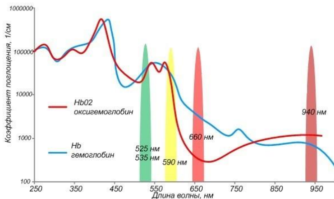
Рис. 1 – График поглощения света кровью и основные спектры излучения пульсовых фотоплетизмографических датчиков [1]
