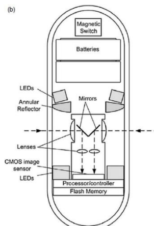
Рис. 3 – Функциональная схема капсулы Capsocam
