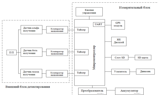
Рис. 1 – Структурная схема устройства для обнаружения и измерения радиоактивного излучения на основе счетчиков Гейгера-Мюллера
