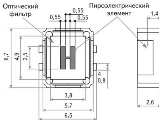
Рис. 2 – Габаритный чертеж пирозлектрического датчика
