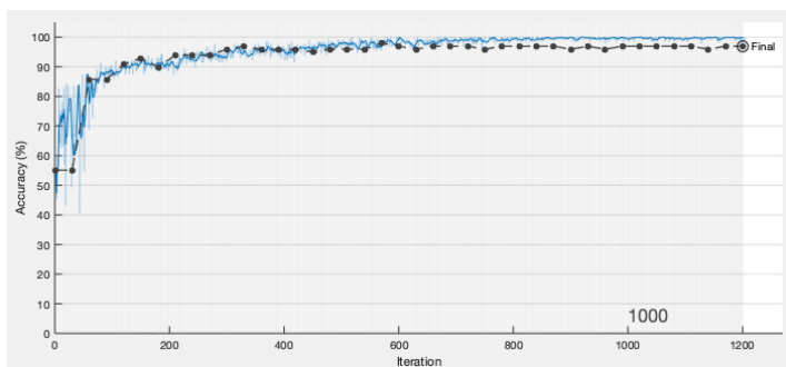
Рис. 3 – График изменения точности при обучении модели
