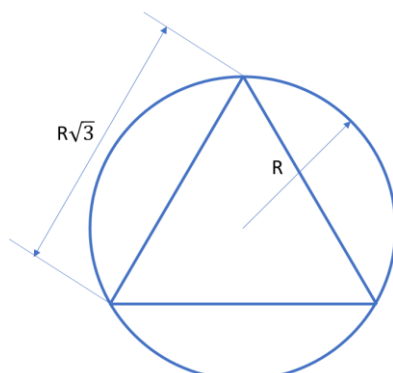
Рис. 6 – Расчет максимальных размеров КМОП матриц в капсуле
