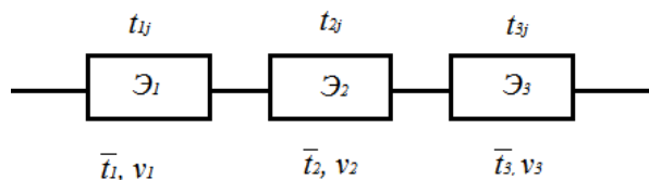
Рис. 1 – Структурная схема невосстанавливаемой нерезервированной последовательной системы
