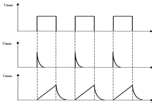
Рис. 2 – Временные диаграммы на различных участках схемы канала воздействия методом электростимуляции
