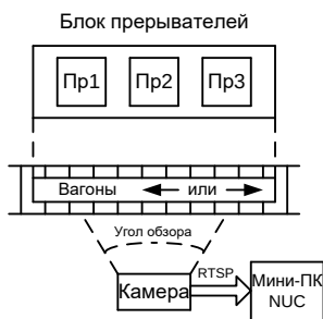
Рис. 1 – структурная схема системы определения направления и скорости движения товарных вагонов
