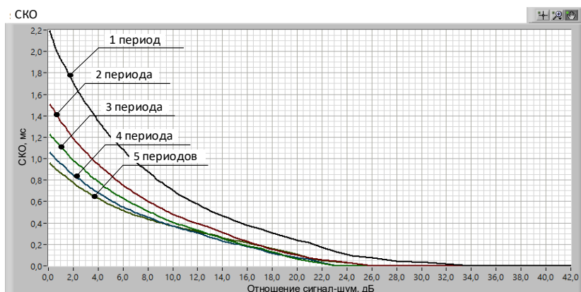
Рис. 1 – Погрешность определения задержки \tau между сигналами
