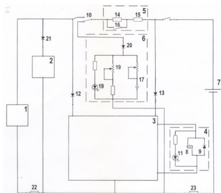
Рис. 2. – Структурно-функциональная схема разработанного устройства
