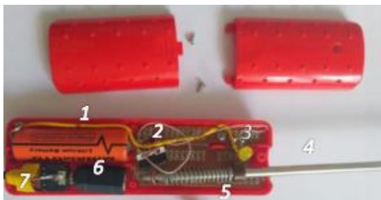
Рис. 2 – Конструкция измерительного электрода. 1 – батарейка номиналом 3 В.; 2 – микропереключатель; 3 – светодиод; 4 – металлический шуп; 5 – пружина; 6 – гнездо; 7 – соединительный контакт
