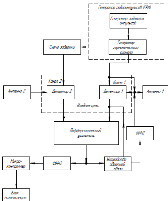
Рис.1 – структурная схема дифференциального радиоимпульсного сенсора
