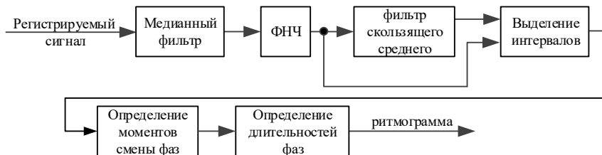
Рис. 3 – Структура процесса цифровой обработки сигнала дыхания
