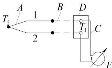
Рис.1 – Схема измерения температуры с помощью термопары A – термопара; B – компенсационный проводник; C – подводящий проводник, D – термостат, E – чувствительный измерительный прибор
