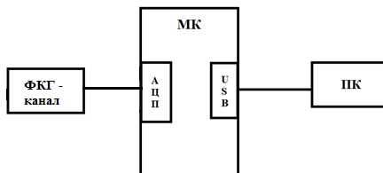
Рис. 2 – Структурная схема системы для оценки параметров фонокардиограммы
