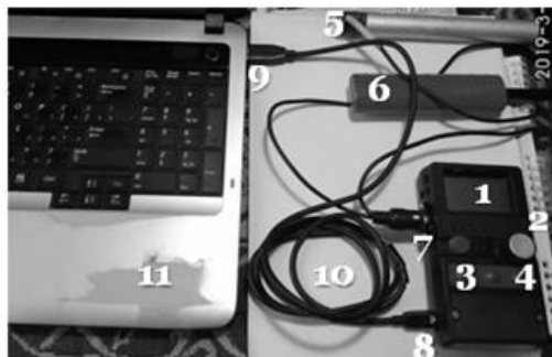
Рис.1 – Конструктивное исполнение комплекса для электропунктурной диагностики: 1 – цифровой микроамперметр; 2 – переключатель питания; 3 – кнопка смены полярности; 4 – потенциометр для регулировки тока; 5 – пассивный электрод; 6 – активный электрод с функцией контроля нажатия на электрод; 7 – разъем для подключения электродов; 8 – вывод microUSB; 9 – вывод USB на ПК; 10 – кабель microUSB; 11 – персональный компьютер (ПК)
