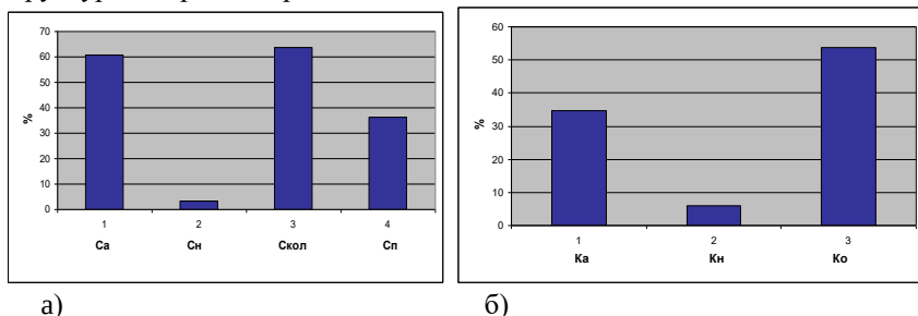
Рис. 1 – Распределение углерода по структурам (а), содержание колец в «средней молекуле» (б)
