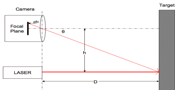
Рис. 1 – Принцип работы триангуляционного лазерного дальномера
