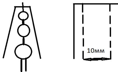
Рис. 3 – Измерительные электроды, копирующие и контактирующие с поверхностью стебля и корня растительного объекта (токоподвод из серебряной или медной фольги показан штрихпунктирной линией)
