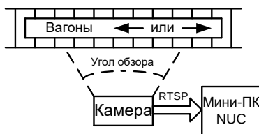
Рис. 1 – Структурная схема системы подсчета количества вагонов товарного поезда с применением зонного детектора движения.
