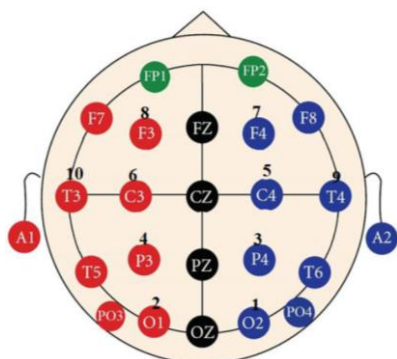
Рис. 1 – Схема расположения электродов
