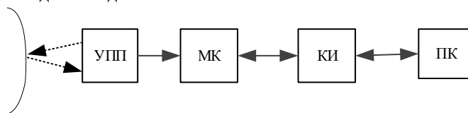
Рис. 2 – Функциональная схема бесконтактного датчика дыхания на основе ультразвуковой эхолокации
