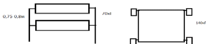
Рис. 2 – Измерительные электроды, копирующие и контактирующие с поверхностью почвы (для измерения u_{ш} расстояние между электродами 0,75-0,8 м, вес по 35 кг)
