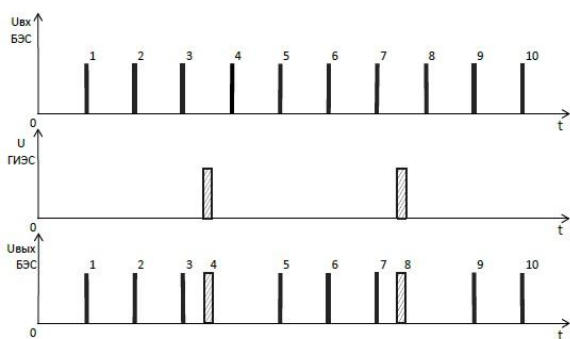
Рис. 2 – Временные диаграммы, демонстрирующие работу блока экстрасистолии
