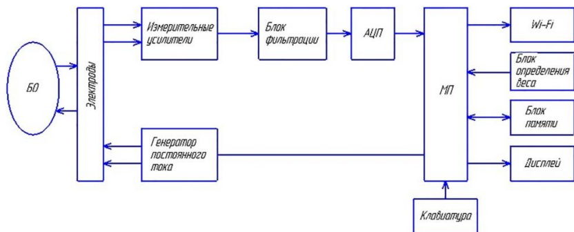
Рис. 1 – Блок-схема анализатора тела
