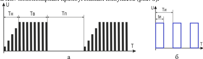
Рис. 3. – Параметры выходного сигнала (абсцисса – T , с; ордината – U , В): а – монополярная последовательность; б – монополярные импульсы ( T_v – время воздействия (1-9 с); T_p – время паузы (0-9 с); T_n – время плавного нарастания сигнала после паузы (0.65 с); t_n – длительность импульса (145 мкс); T_n – период следования импульсов ( F=1/T_n , 40-400 Гц))
