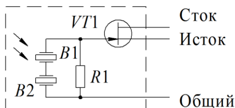
Рис. 1 – Типовое схемотехническое исполнение пирозлектрического датчика 4
