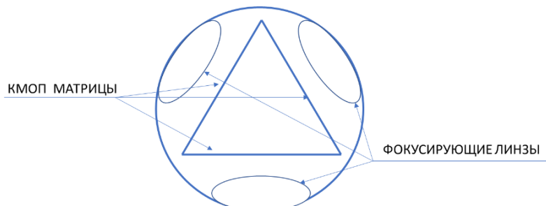
Рис. 5 – Расположение КМОП матриц внутри капсулы (вид с торца)
