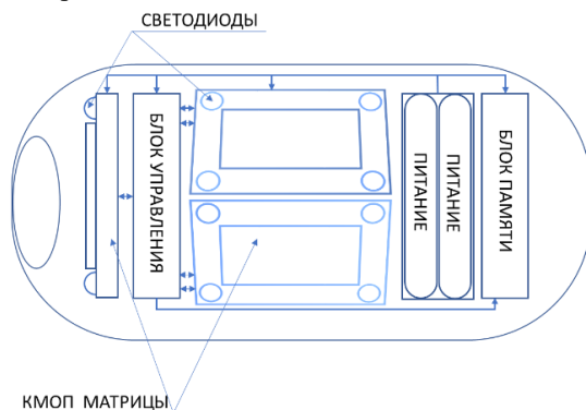
Рис. 4 – Функциональная схема видеокапсулы
