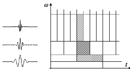
Рис.1 – Пример вейвлетов при различных масштабах и их схематичные изображения в плоскости время-частота
