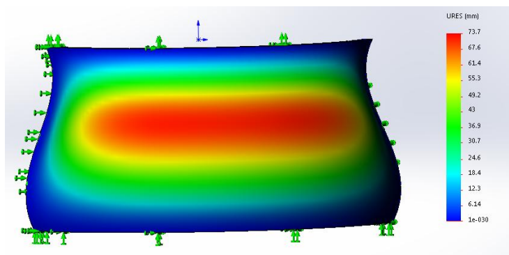
Рисунок 1 – Эпюра перемещений при давлении 14 мм рт ст
