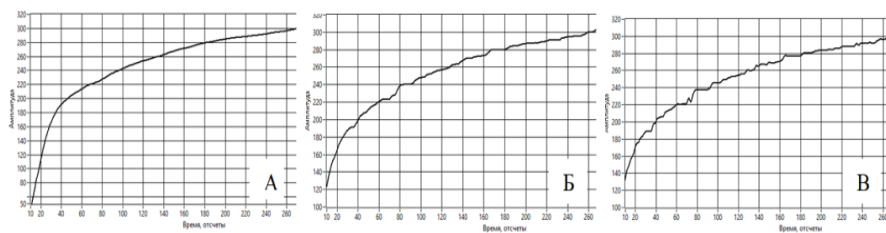
Рис. 3 – Графики отфильтрованного сигнала с использованием фильтров Баттерворта (А), Бесселя (Б) и Чебышева (В)
