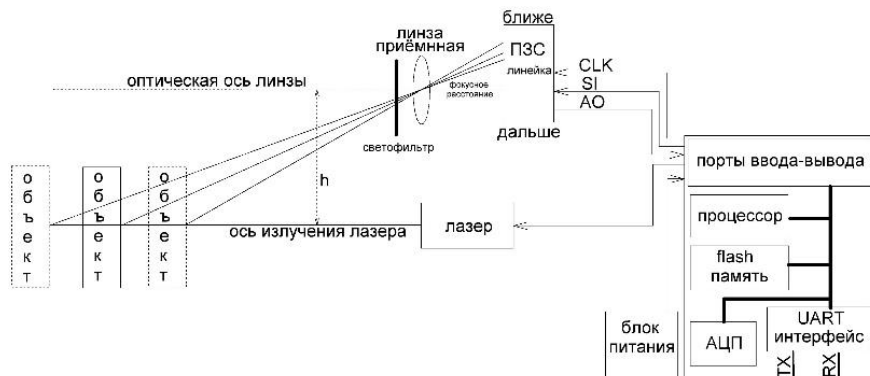
Рис. 2 – Функциональная схема триангуляционного лазерного дальномера
