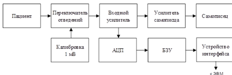
Рис. 1 – Структурная схема электрокардиографа
