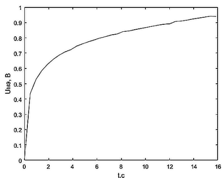
Рис.1 – График зависимости межэлектродного напряжения от времени
