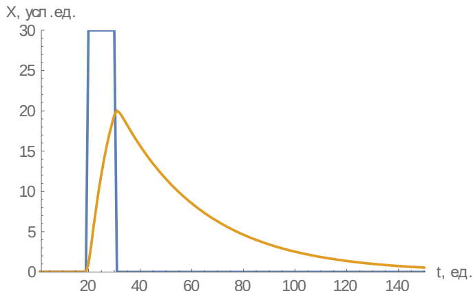
Рис. 2 – График воздействия входной величины и отклика датчика
