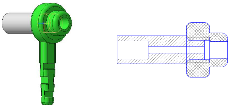
Рис.2 – Конструктивный вариант корпуса электрода для проведения термокартирования
