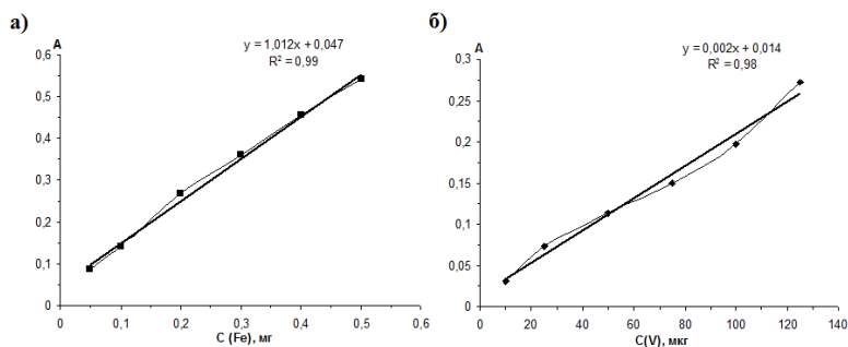
Рис. 1 – Градуировочный график для определения железа (а) и ванадия (б)
