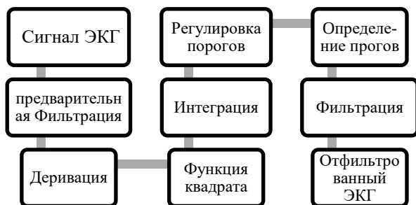
Рис. 2 – Шаги для анализа сигнала ЭКГ
