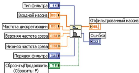
Рис. 2 – Блок-диаграмма фильтра Баттерворта в Labview
