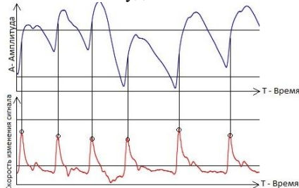
Рис. 2 – Производная полученного ФПГ сигнала и выделение максимальных точек
