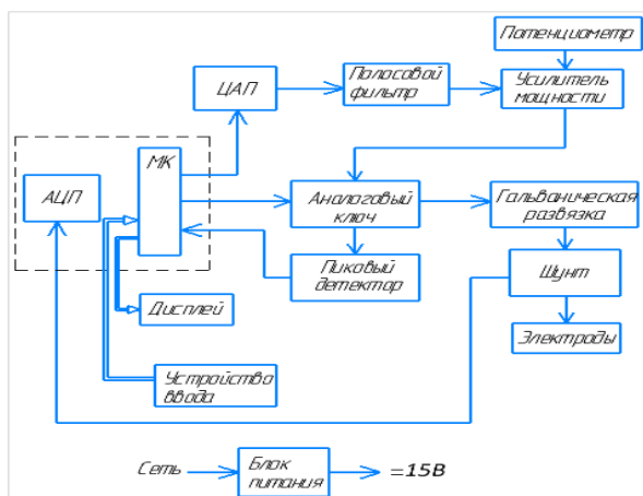
Рис. 1 – Структурная схема разрабатываемого устройства
