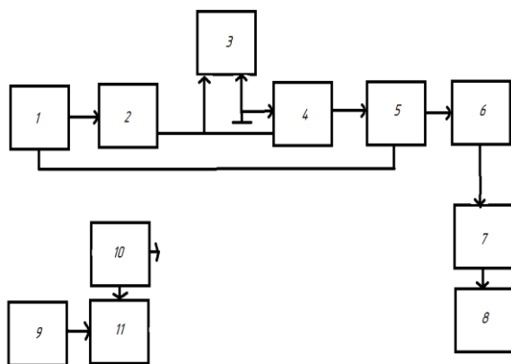
Рис.1. – Структурно-функциональная схема измерителя параметров кожных новообразований:
