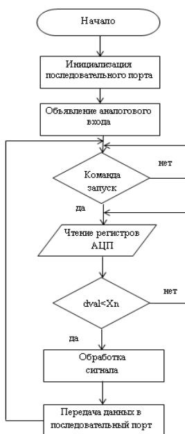
Рис.3 – Алгоритм ПО
