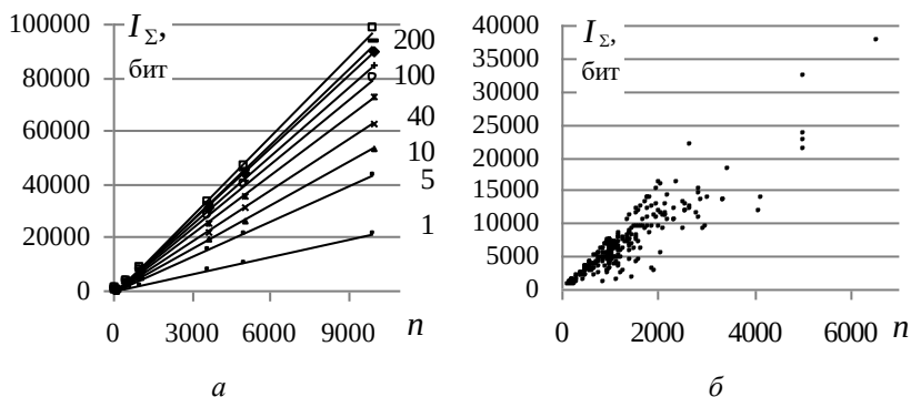
Рис. 1 – Графические диаграммы: I_{\Sigma}(n, \sigma) для ВРВП (а), I_{\Sigma}(n) для ВРРП ритма сердца разных групп здоровых и больных людей (б)
