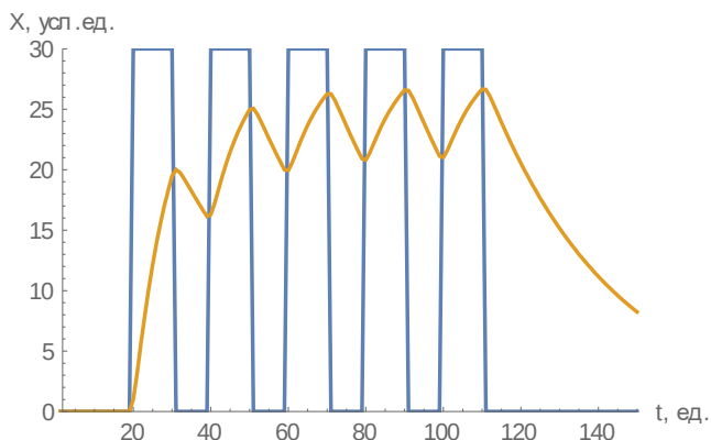
Рис. 3 – Отклик датчика при многократном воздействии газа
