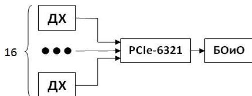
Рис.1 – Элементы системы контроля магнитного поля
