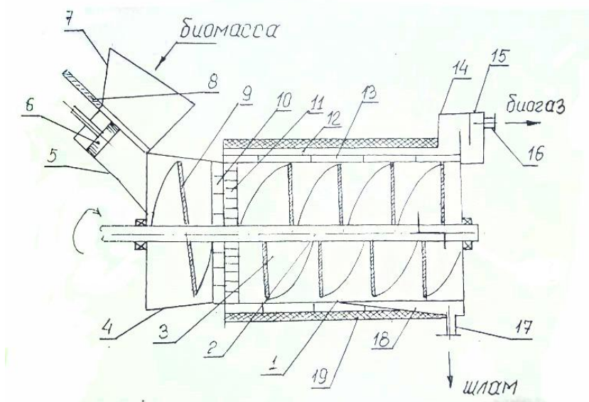
Рис.1 – Схема биореактора
